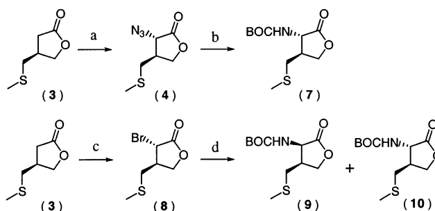
Scheme 3. (a) LiHMDS, -78^{\circ}\text{C} ; Tris-N 3 then HOAc 45%; (b) SnCl 2 or PPh 3 , H 2 O; BOC 2 O, 80%; (c) LiHMDS, -78^{\circ}\text{C} ; NBS, THF, 48%; (d) TMGA, CH 2 Cl 2 ; PPh 3 , H 2 O, THF; BOC 2 O, 60% (1.3:1).
